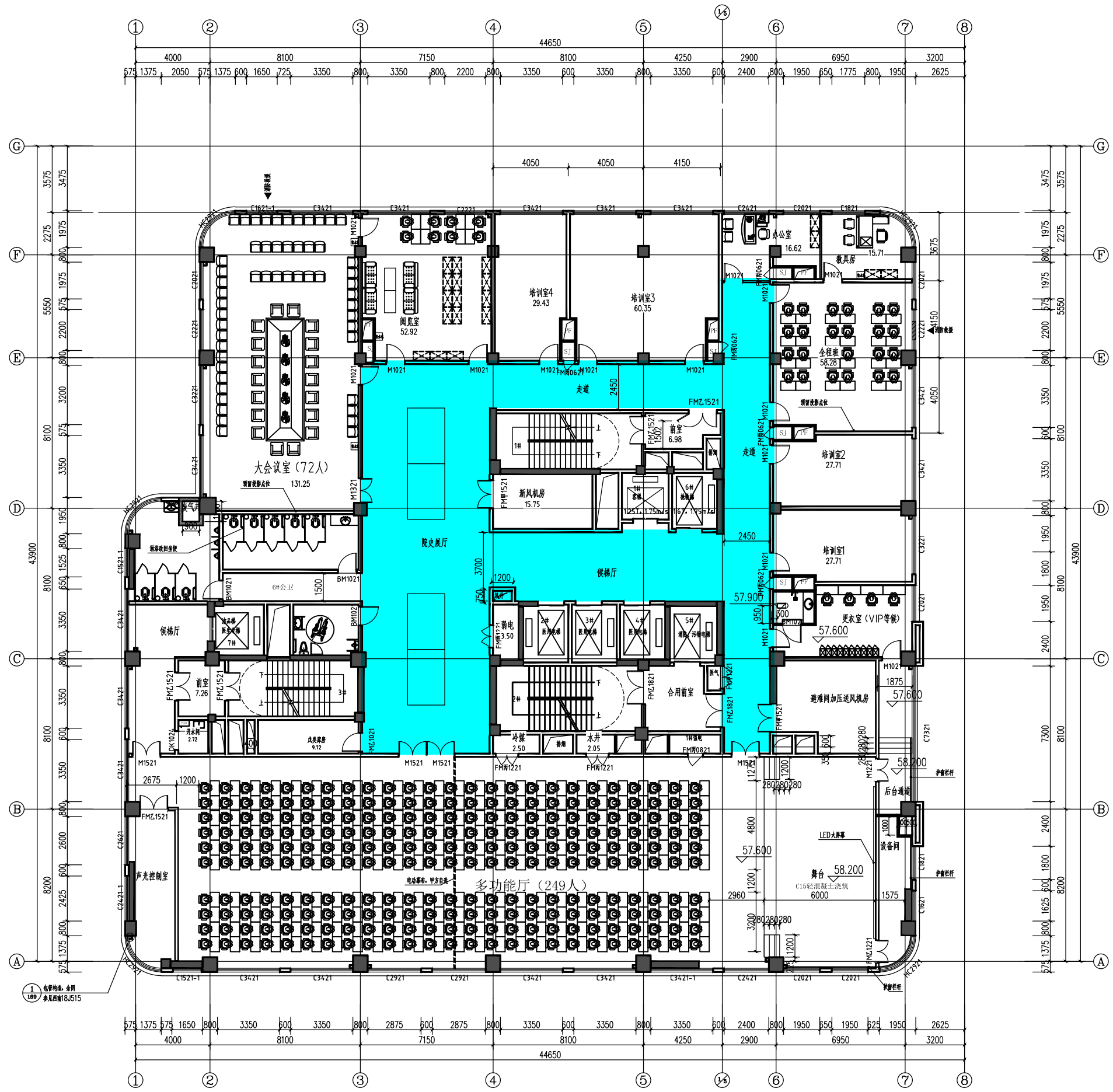
十五层平面图 1:100
